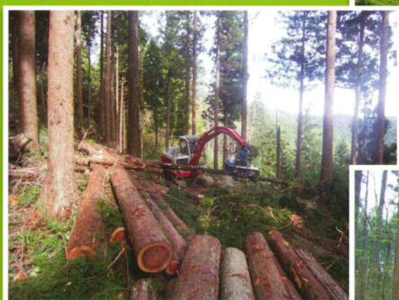
高性能林業機械による造材
