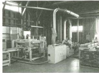
フィンガージョイント加工機
